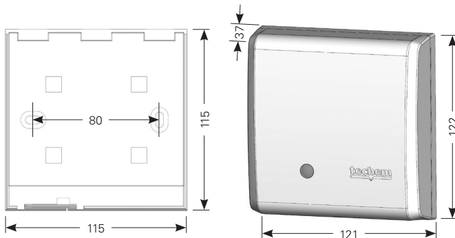
Wandmontageplatte
